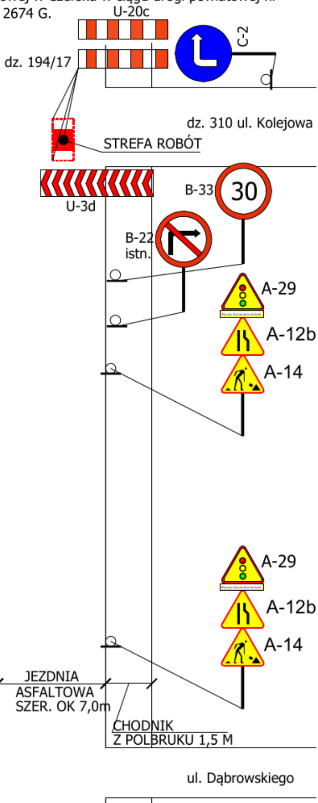
SCHEMAT NR 1 OZNAKOWANIA ROBÓT NA CZAS PROWADZENIA PRAC BUDOWLANYCH B/S
